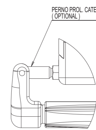
DETTAGLIO D SCALA 1:1
